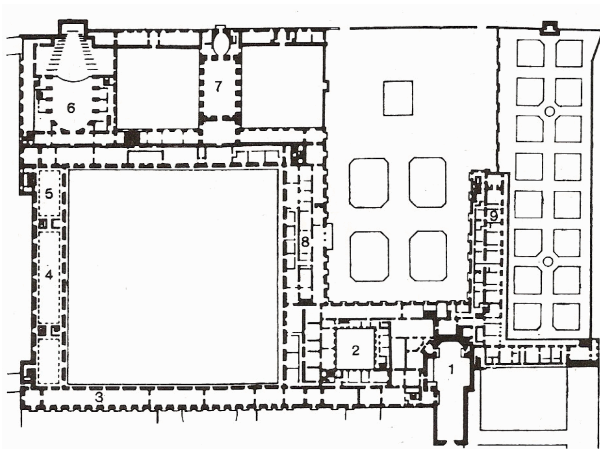
Floor plan of Buen Retiro Royal Palace in 1640. Number 4, Hall of Realms (J. Brown y J.H. Elliot, 1980).
